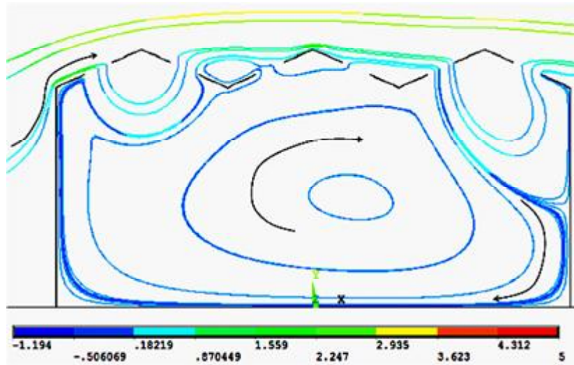
Figura 12. Líneas de trayectoria del aire del escenario 4 (modelo completo).
