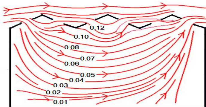
Figura 13. Líneas de trayectoria y velocidades ( \text{m s}^{-1} ) del aire del escenario 4 (modelo simplificado).
