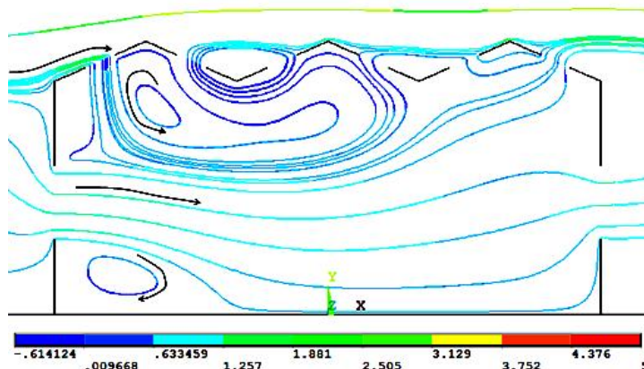
Figura 14. Líneas de trayectoria del escenario 5 (modelo completo).
