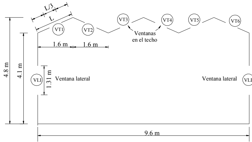
Figura 2. Sección transversal del invernadero de estudio tipo Venlo.
