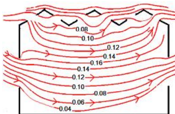
Figura 15. Líneas de trayectoria y velocidades ( m s^{-1} ) del escenario 5 (modelo simplificado).
