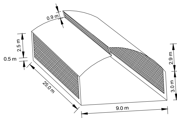
Figura 1. Invernadero utilizado para la calibración del modelo de Navier-Stokes completo.
