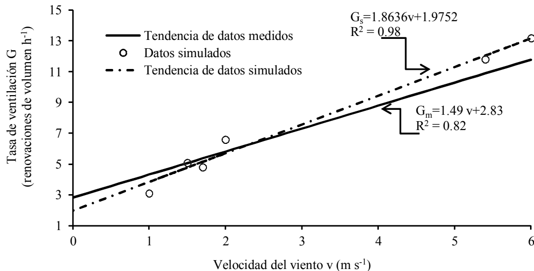
Figura 7. Datos medidos y simulados de tasas de ventilación, bajo ventilación lateral del invernadero experimental.
