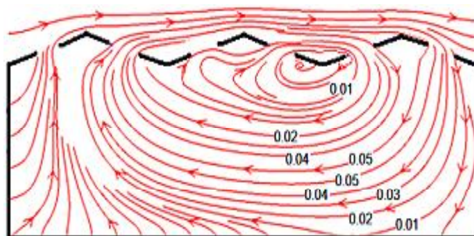
Figura 11. Líneas de trayectoria y velocidades ( \text{m s}^{-1} ) del aire del escenario 3 (modelo simplificado).
