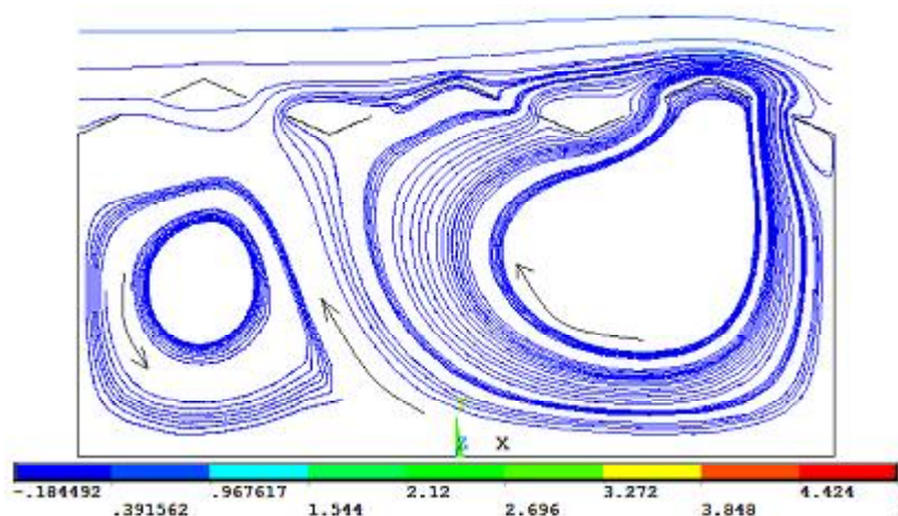
Figura 10. Líneas de trayectoria del escenario 3 (modelo completo).
