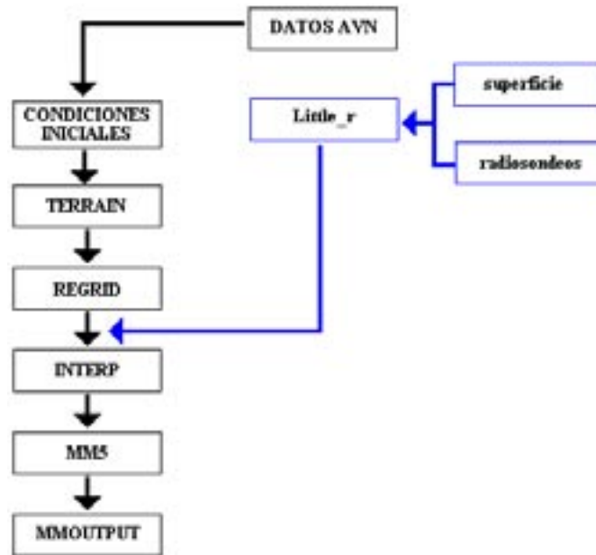
Figura 1. Esquema del sistema de automatización del modelo MM5, este sistema funciona diariamente partiendo en su estado actual con las conexiones vía ftp a un servidor que concentra la mayoría de los resultados de los modelos numéricos tanto de área limitada como de escala global, en una etapa próxima (color azul) se implementará la asimilación de datos obtenidos por la red nacional de observatorios meteorológicos y de radiosondeos.
