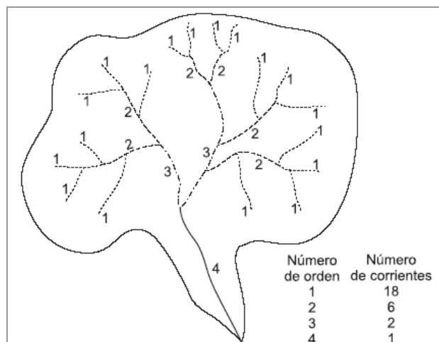
Figura 6. Ordenación de cauces de acuerdo al criterio de Horton - Strahler
